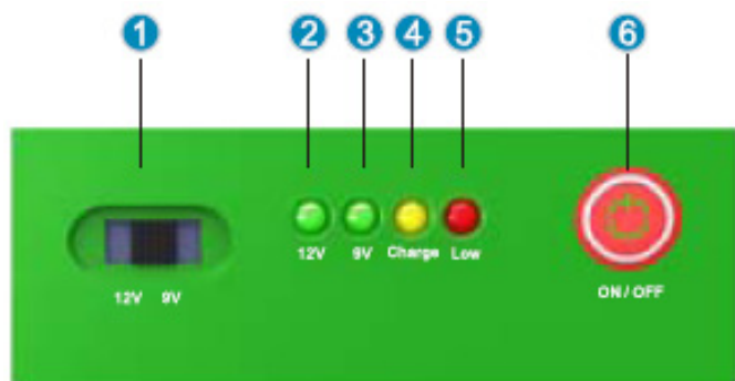
Descrizione pannello frontale
